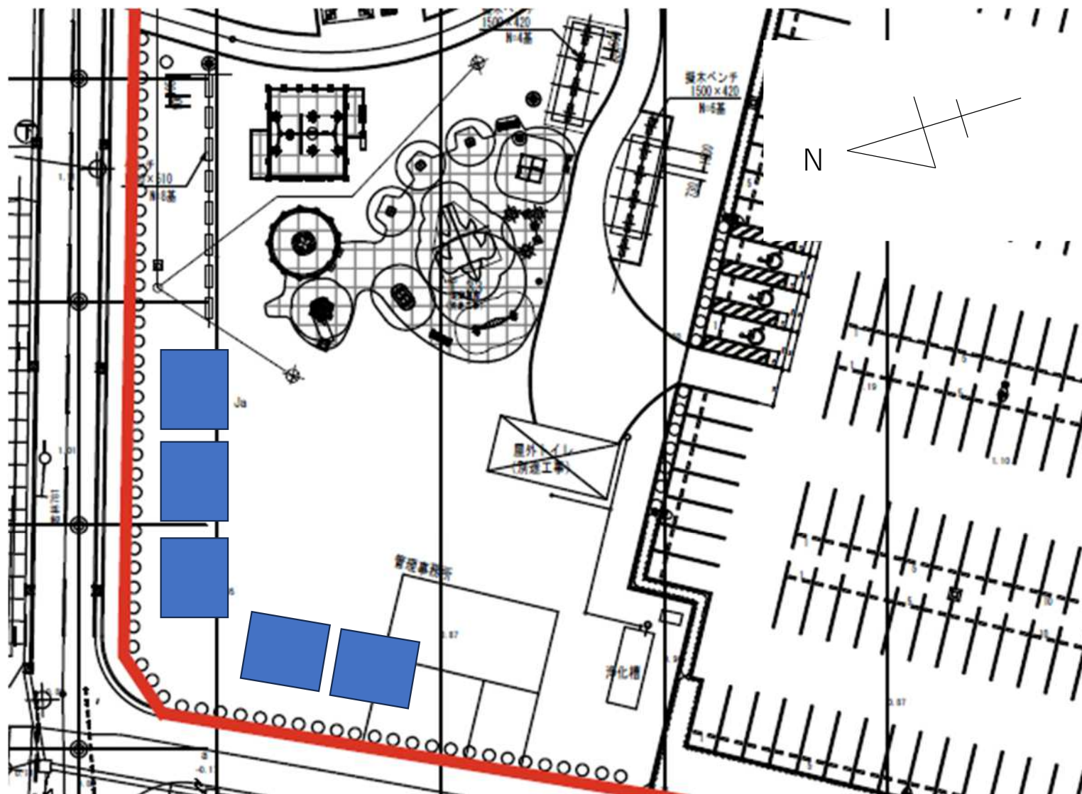
詳細図
